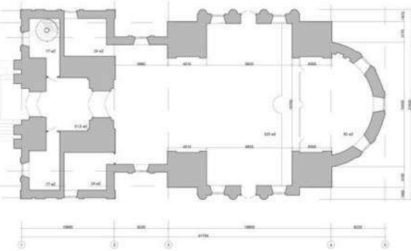
План на отн. 0.000
