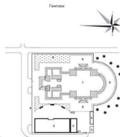
Генплан
