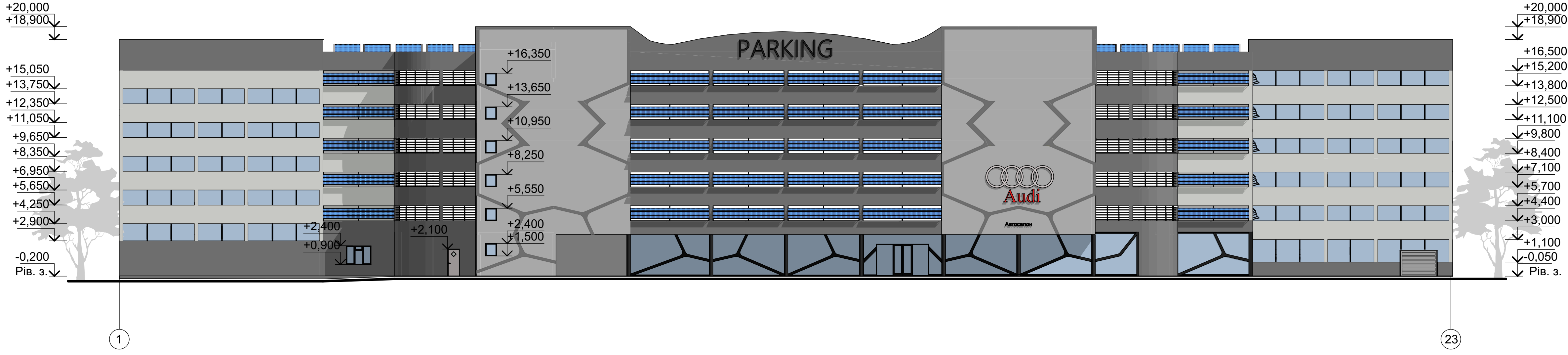
Фасад 1-23 М 1:200
