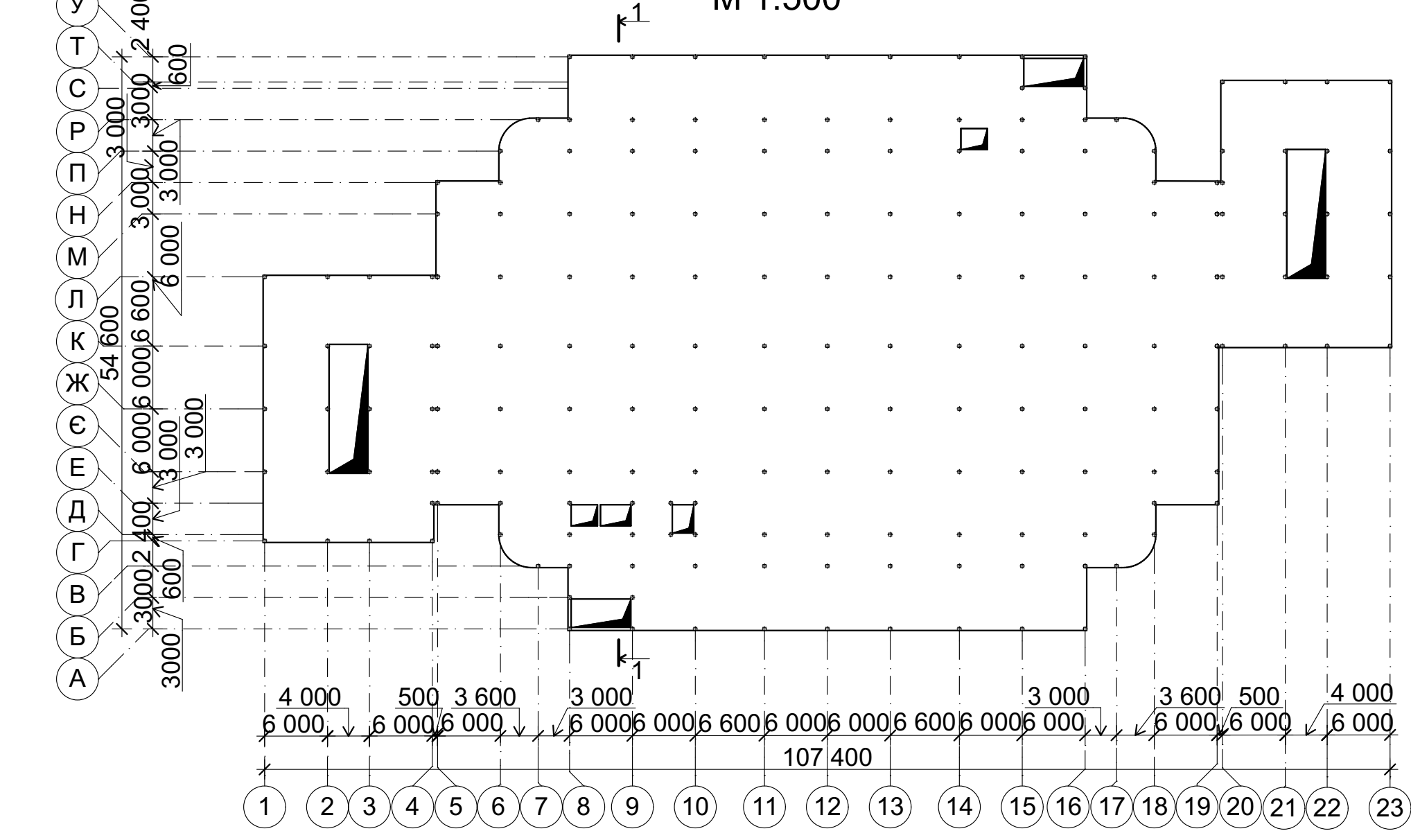
Схема розташування елементів перекриття М 1:500
