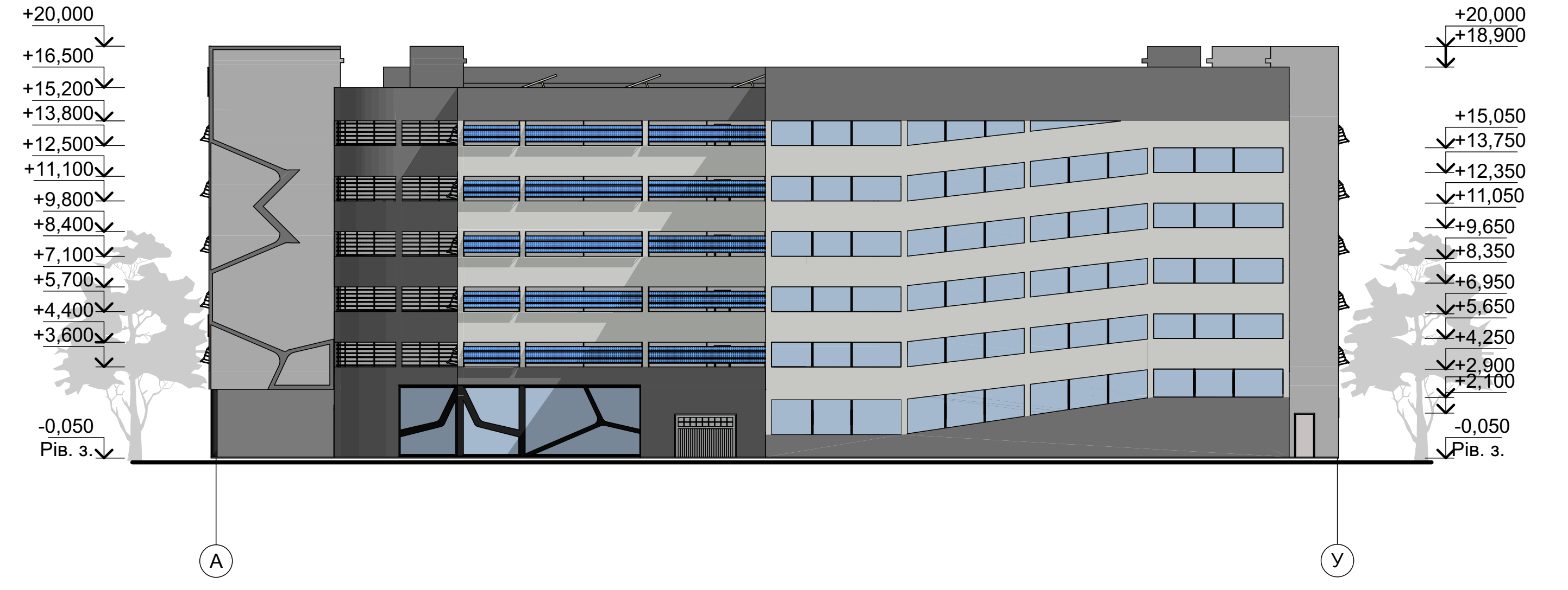
Фасад П-А М 1:200
