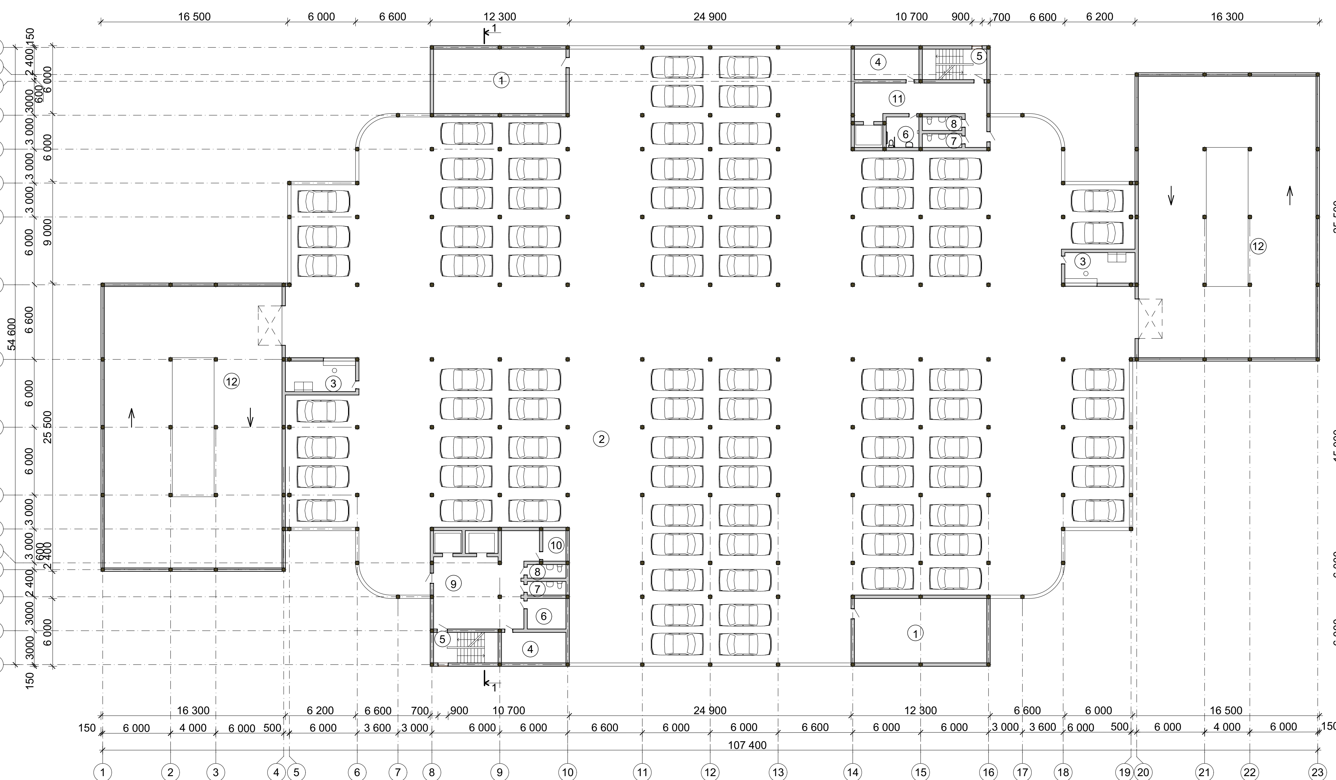
План на відм. +3,600,....+14,400 М 1:200
