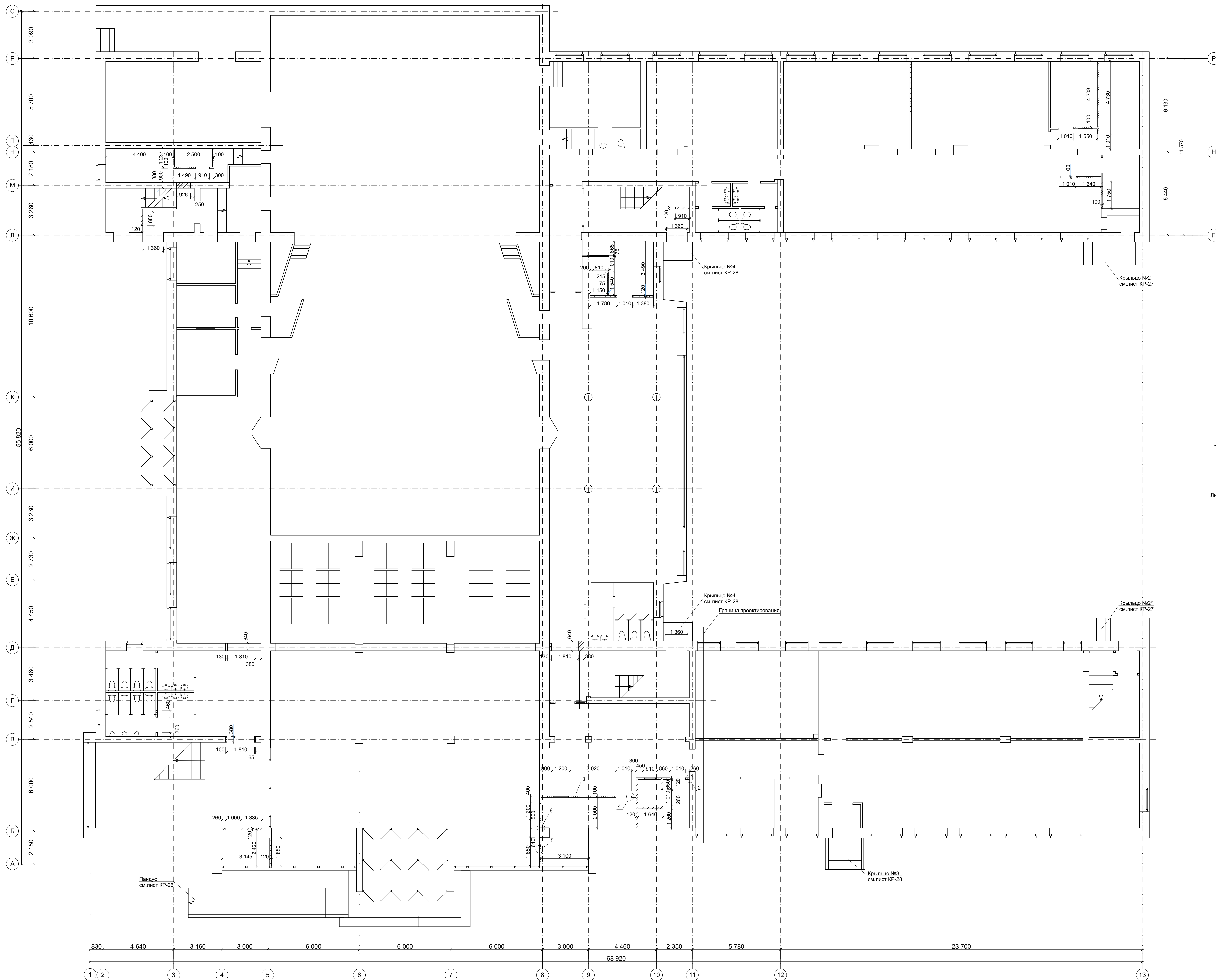
Кладочный план на отм. 0.000 М 1:100.
