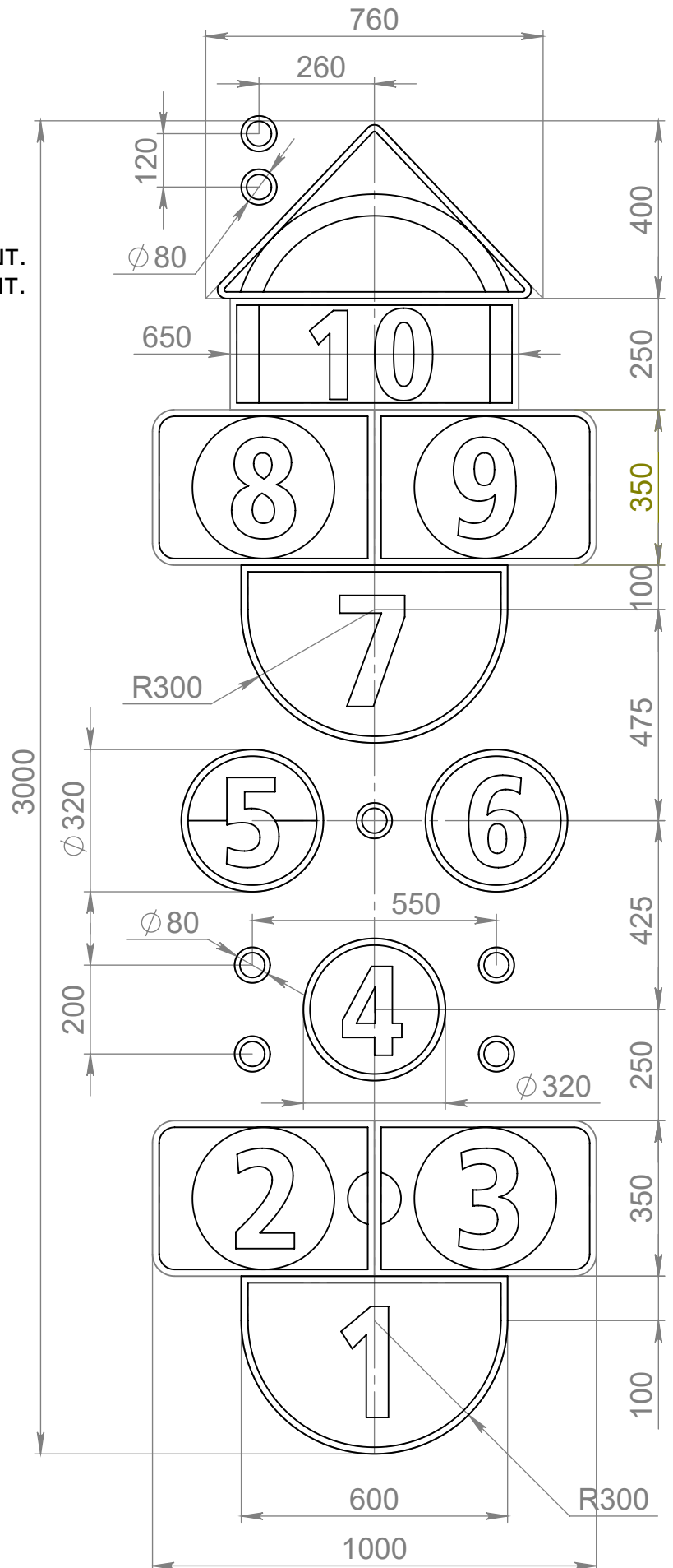
Схема расположения плит
